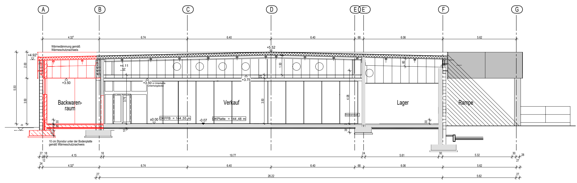
Schnitt A-A
